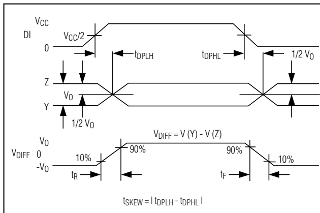
图3. 驱动器传输延时
