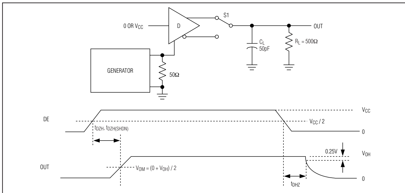
图4. 驱动器使能和禁用时序( t_{DZH} 、 t_{DZH(SHDN)} )
