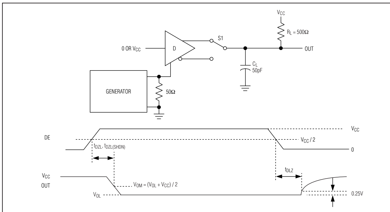
图5. 驱动器使能和禁用时序( t_{DLZ} 、 t_{DLZ(SHDN)} )
