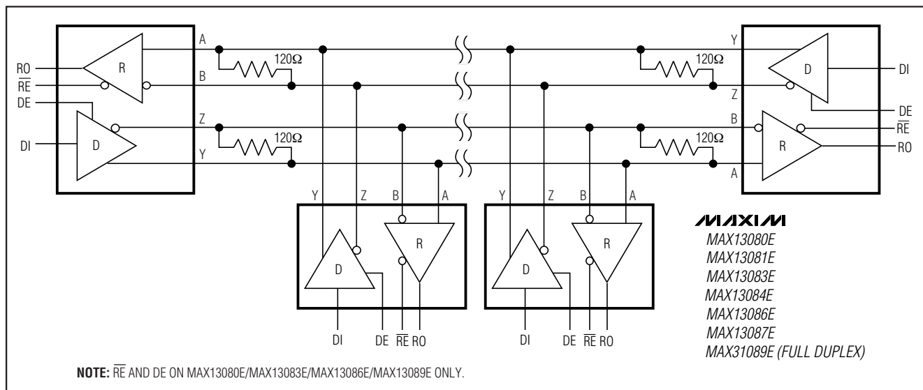
图13. 典型全双工RS-485网络
